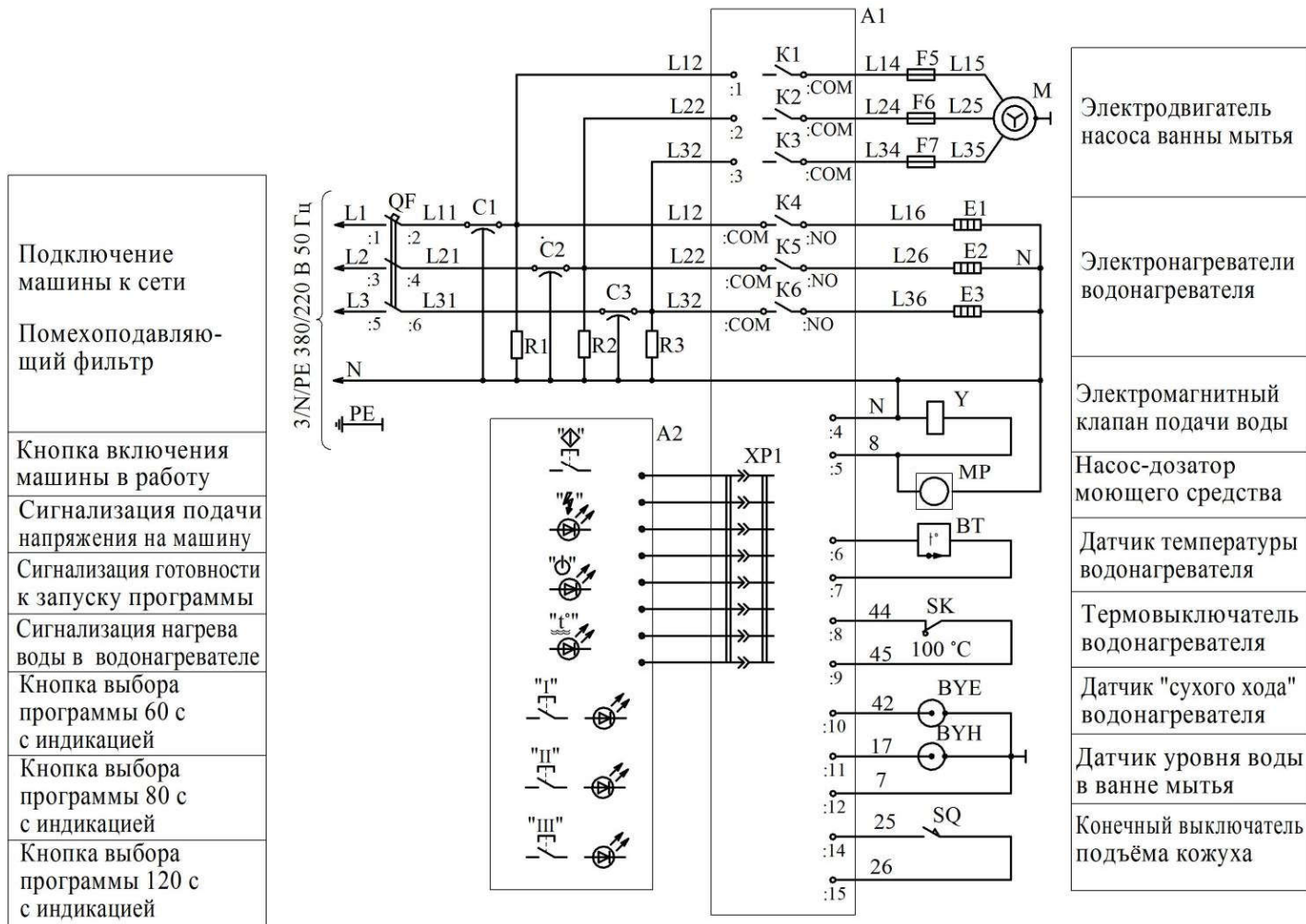
Рисунок 3 – Схема электрическая принципиальная
