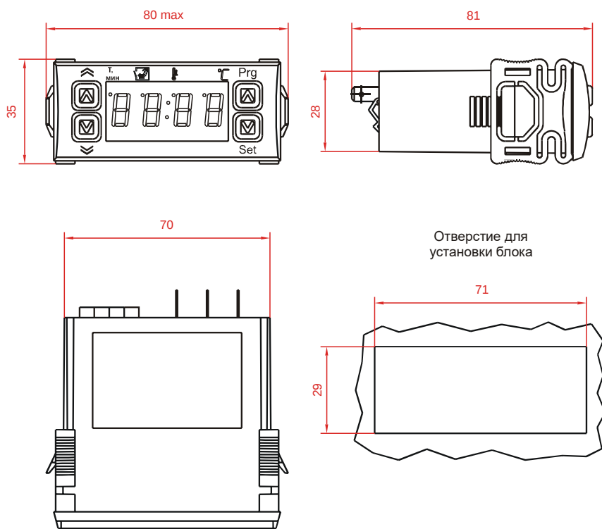
Рис 1 Габаритные размеры блока (размер окна для установки блока - 71x29 мм)
