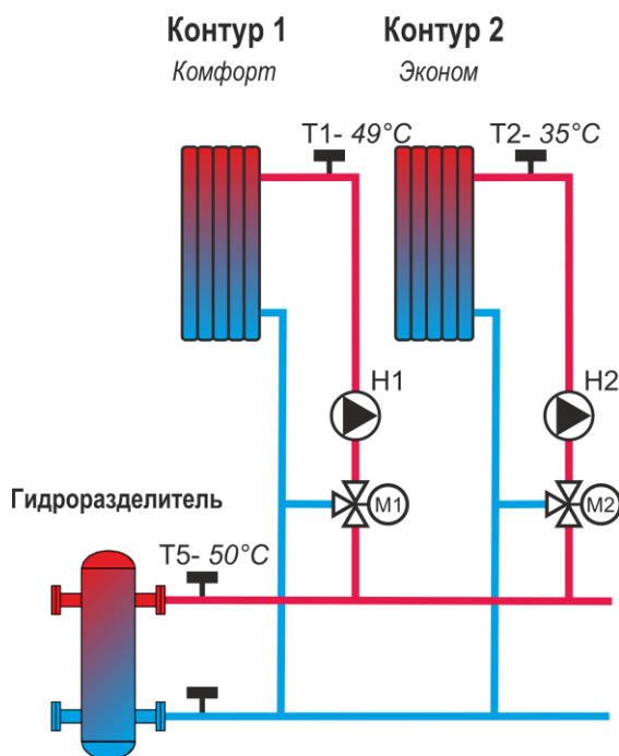
Рисунок 4 Управление контуром отопления
