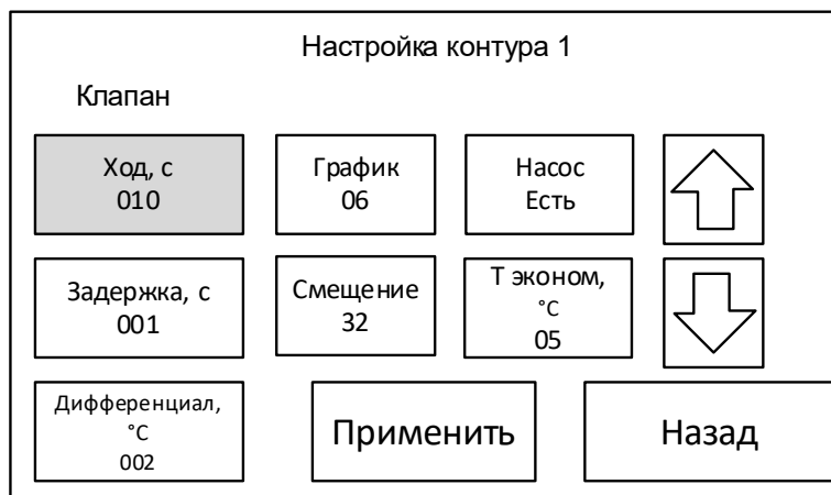
Рисунок 10 Настройка параметров контура отопления
