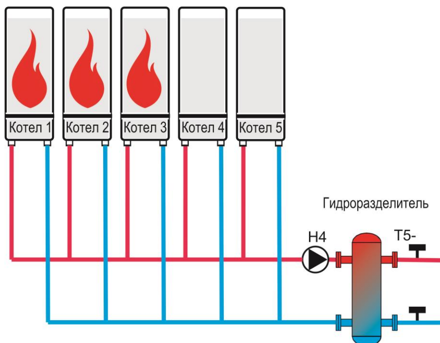
Рисунок 3 Управление каскадом котлов
