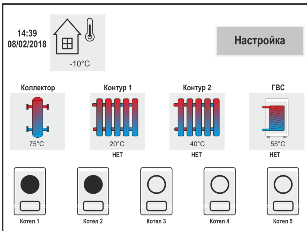
Рисунок 13 Главный экран программы при первом включении
