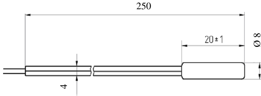
Рисунок 16 Габаритные и установочные размеры датчика наружной температуры T5.
