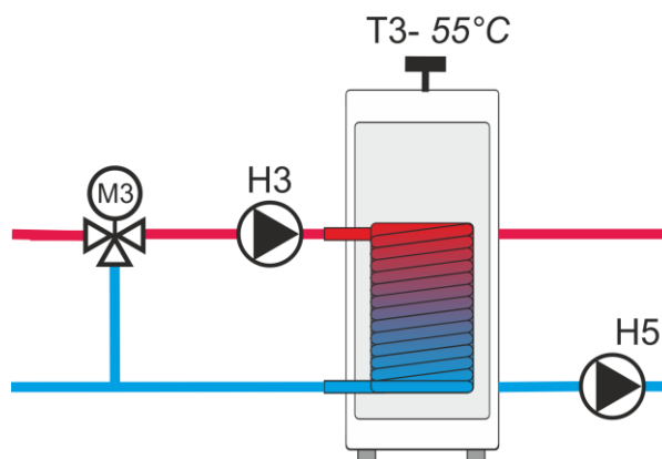
Рисунок 5 Управление контуром ГВС
