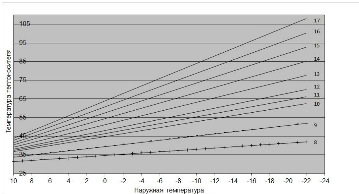
Рисунок 20 График погодозависимости для радиаторного отопления
