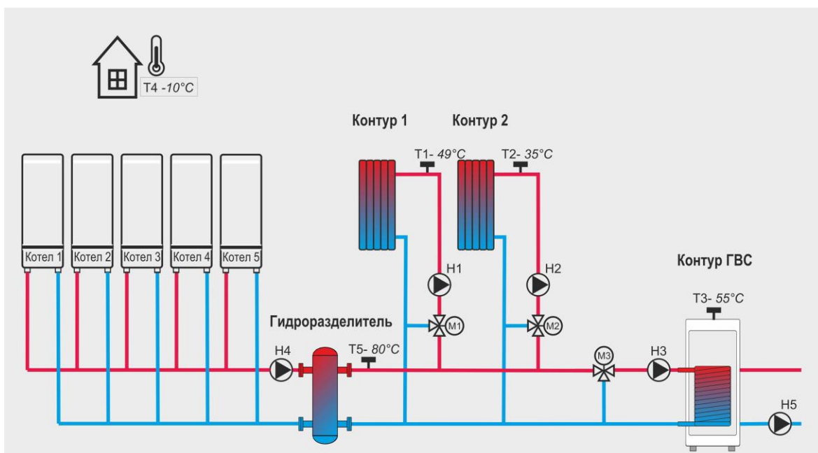
Рисунок 1 Функциональная схема котельной
