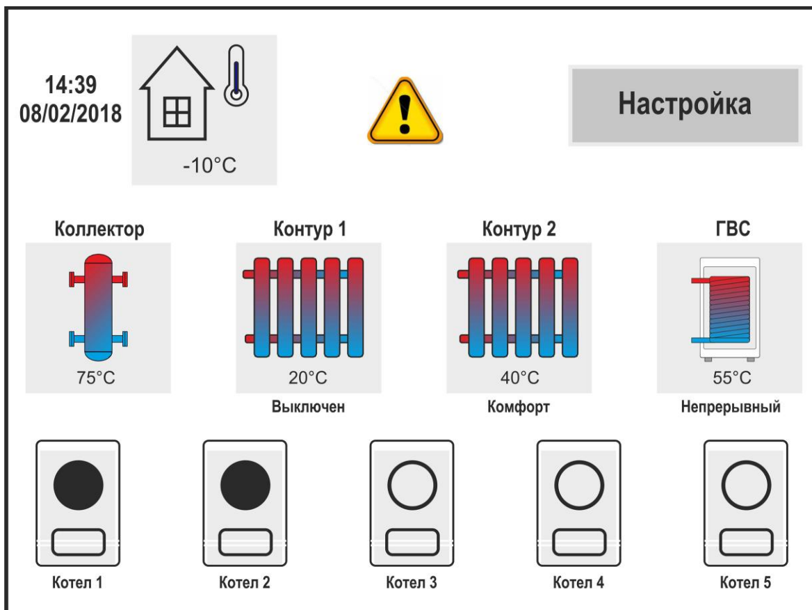
Рисунок 2 Главный экран программы
