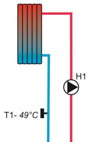
Рисунок 12 Контур отопления, управляемый только насосом
