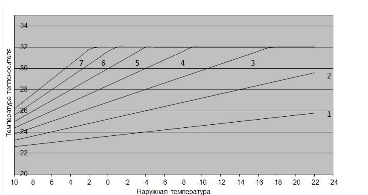
Рисунок 21 График погодозависимости для теплого пола
