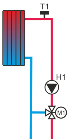
Рисунок 11 Контур отопления, управляемый 3-х ходовым клапаном и насосом
