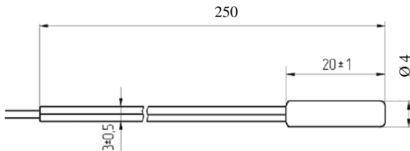
Рисунок 17 Габаритные и установочные размеры датчиков температуры теплоносителя (T1-T4).
