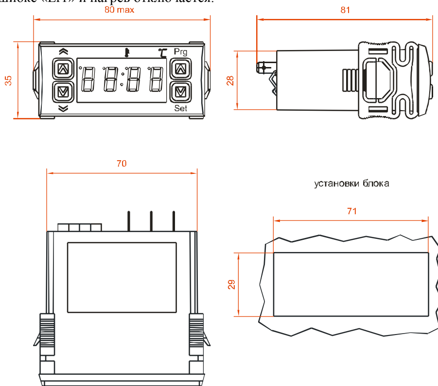
Рисунок 1. Внешний вид, габаритные и установочные размеры блока.
