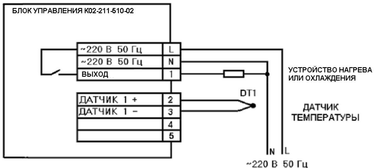
Рисунок 3. Схема электрического подключения блока в составе оборудования
