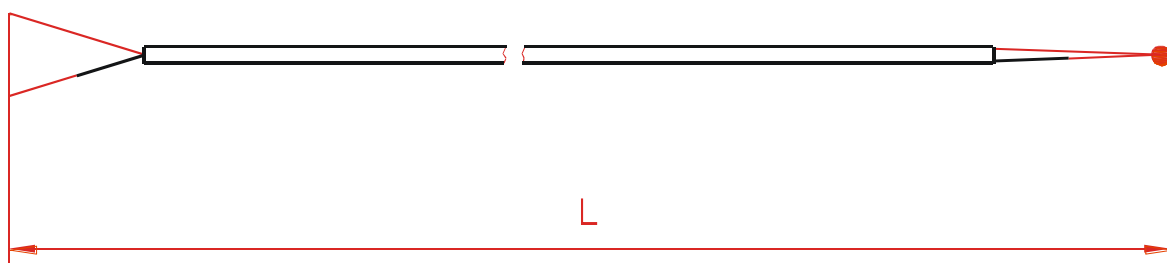
Рисунок 2. Внешний вид и габаритные размеры датчика температуры исполнения Т на термопаре ТХЛ (L) по СТБ ГОСТ Р 8.585.
